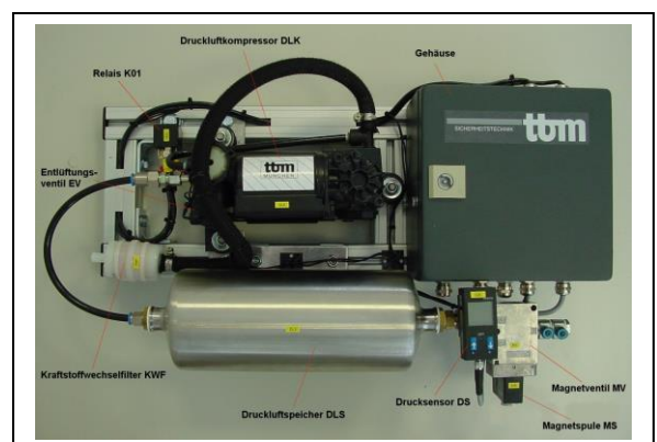
Luftduschen-Kompressor-Einheit
